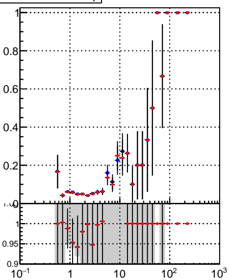
■ tracking_Iters01LST_10evt_CPU ■ tracking_Iters01LST_10evt_GPU
