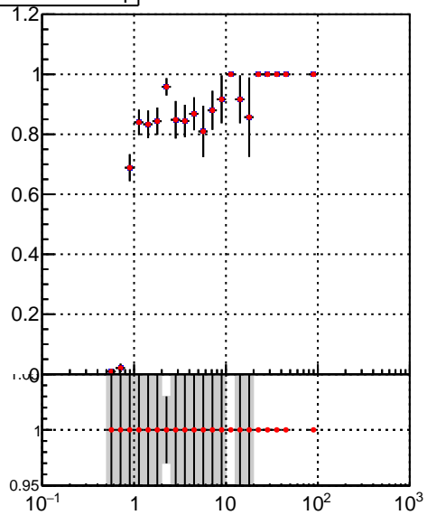
■ tracking_Iters01LST_10evt_CPU ■ tracking_Iters01LST_10evt_GPU
