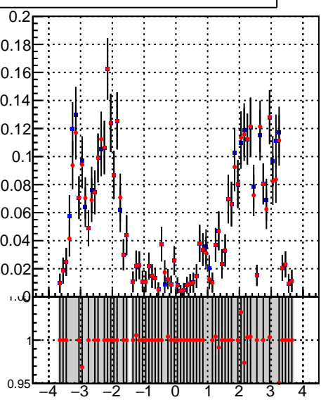
■ tracking_Iters01LST_10evt_CPU ■ tracking_Iters01LST_10evt_GPU
