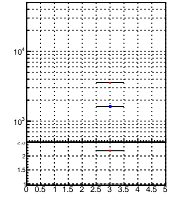
pix layer
