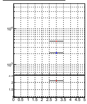
oob trackingLST-rmIS-mask-8c1d76e
