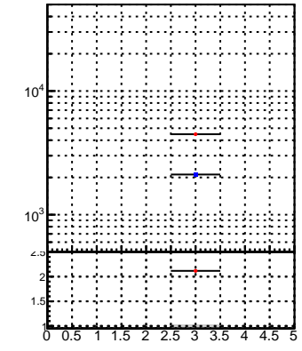
oob trackingLST-rmIS-mask-8c1d76e
