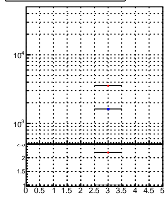
pix layer
