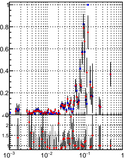
—●— oob —●— trackingLST-rmIS-mask-8c1d76e
