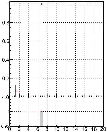
Fake rate vs. oob trackingLST-rmIS-mask-8c1d76e
