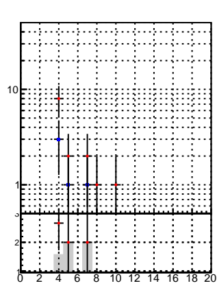
—●— oob —+— trackingLST-rmIS-mask-8c1d76e
