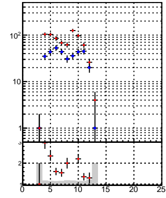
—●— oob —+— trackingLST-rmIS-mask-8c1d76e
