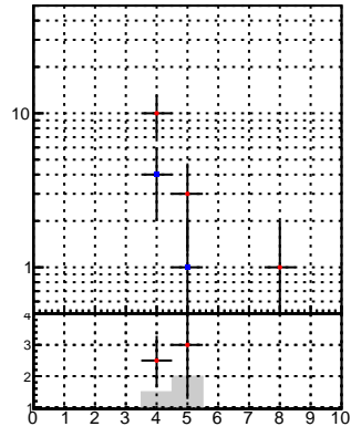
—●— oob —+— trackingLST-rmIS-mask-8c1d76e
