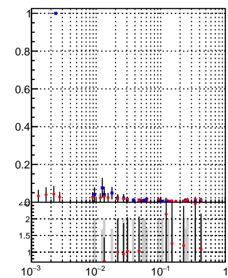
Fake rate vs \tau oob trackingLST-rmIS-mask-8c1d76e
