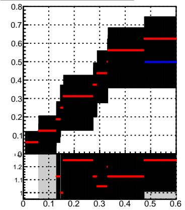
Fake rate oob trackingLST-rmlS-mask-8c1d76e
