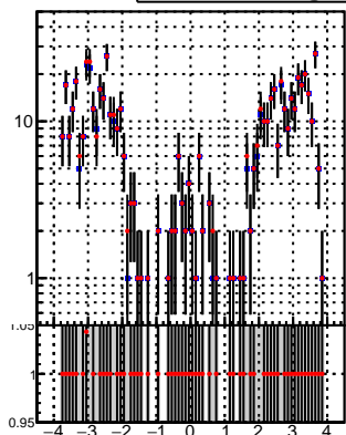
—●— oob —●— trackingLST-rmlS-mask-8c1d76e
