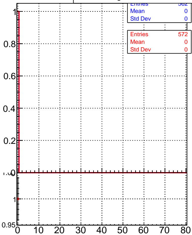
oob trackingLST-rmIS-mask-8c1d76e
