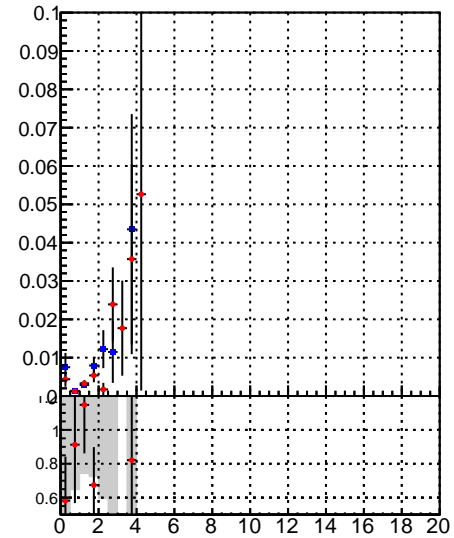
Fake rate vs. oob trackingLST-rmIS-mask-8c1d76e
