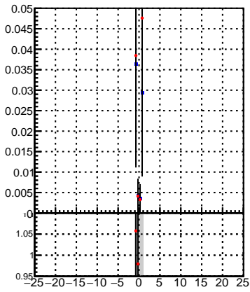
oob trackingLST-rmlS-mask-8c1d76e
