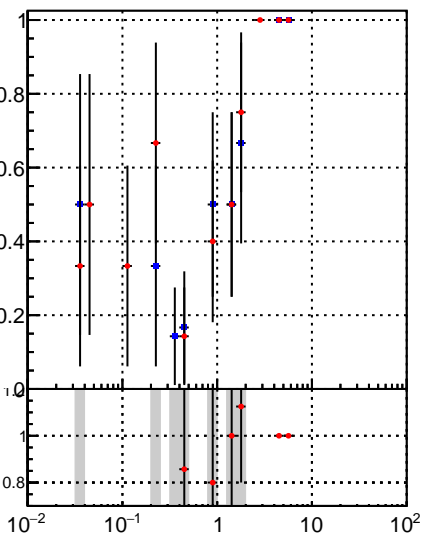
Fake rate vs \nu —■— oob —●— trackingLST-rmIS-mask-8c1d76e
