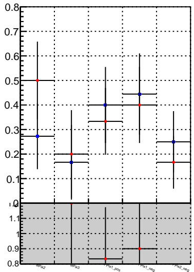
Fake rate vs. —♦— oob —●— trackingLST-rmIS-mask-8c1d76e
