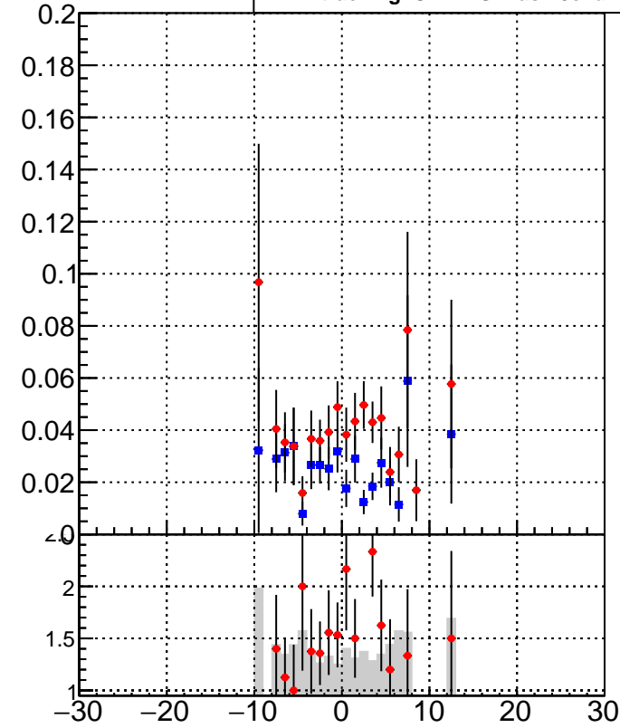
■ oob ● trackingLST-rmIS-mask-8c1d76e
