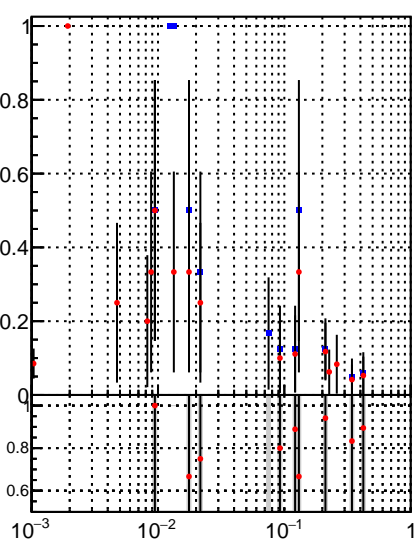
Fake rate vs pu oob trackingLST-rmIS-mask-8c1d76e
