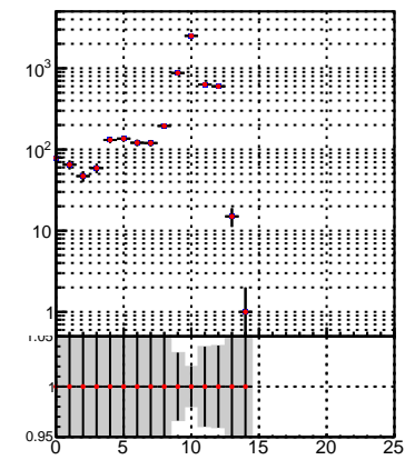
—●— oob —●— trackingLST-rmIS-mask-8c1d76e
