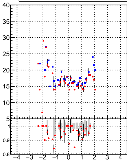
mean hit oob trackingLST-rmlS-mask-8c1d76e
