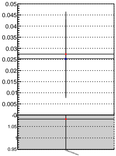
Fake rate vs. oob trackingLST-rmIS-mask-8c1d76e
