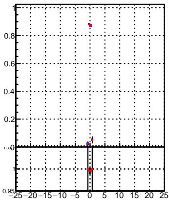
Efficiency ■ oob ■ trackingLST-rmIS-mask-8c1d76e
