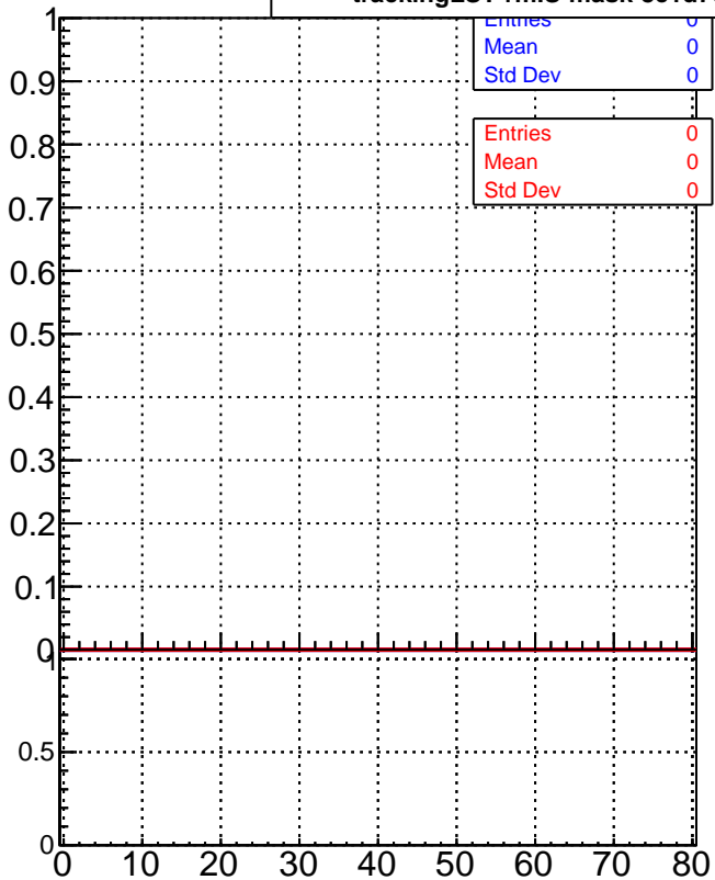
oob trackingLST-rmIS-mask-8c1d76e
