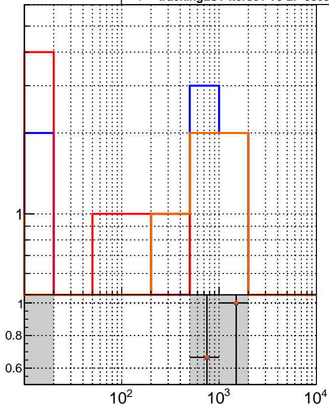
RecoAssoc2GenPV
