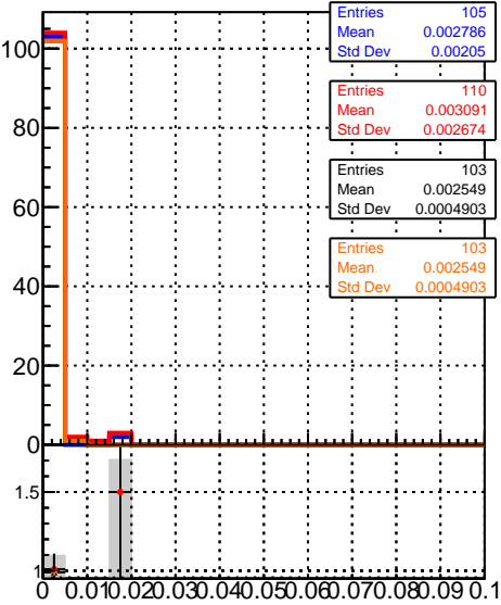
Recons trackingIters01-03fac7e oob trackingLST-Iters01-03fac7e trackingLST-Iters01-T5-2P-33e94a6
