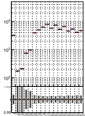
N of reco track vs. \chi^2 trackingIter01-03fac7e trackingLST-Iter01-03fac7e trackingLST-Iter01-15-2P-33e94a6
