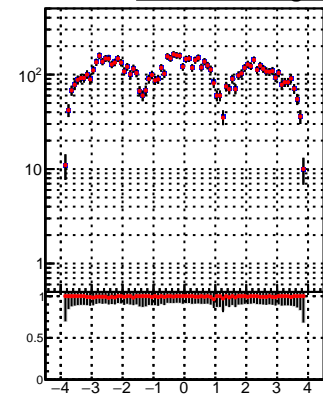
N of reco track vs eta trackingLST-Iter01-03fac7e trackingLST-Iter01-03fa67e trackingLST-Iter01-03fa67e-15-2P-33e94a6
