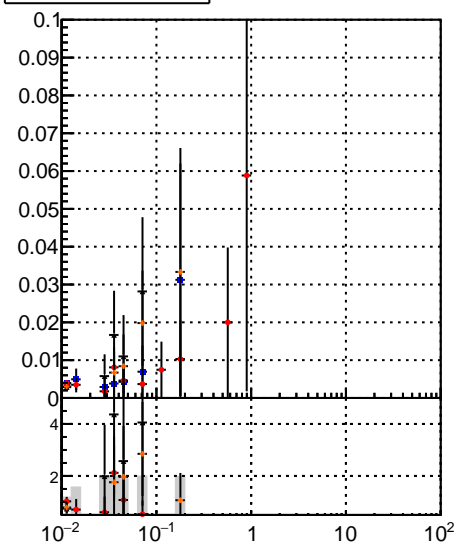
trackingITers01-03fac7e OOB trackingLST-ITers01-03fac7e trackingLST-ITers01-T5-2P-33e94a6
