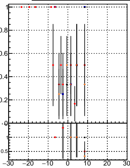
■ trackingITers01-03fac7e ■ 00b ■ trackingLST-ITers01-03fac7e ■ trackingLST-ITers01-T5-2P-33e94a6
