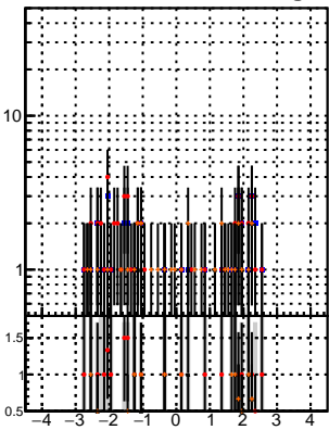
N of reco track vs \eta — trackingLST-Iter01-03fac7e — trackingLST-Iter01-03fac7e — trackingLST-Iter01-03fac7e — trackingLST-Iter01-03fac7e
