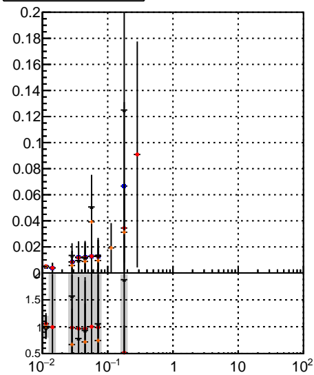
■ trackinglters01-03fac7e ■ oob ■ trackingLT-lters01-03fac7e ■ trackingLT-lters01-T5-2P-33e94a6
