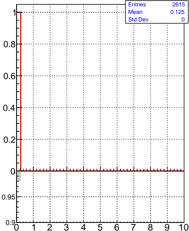
dE/dx estimator 1
