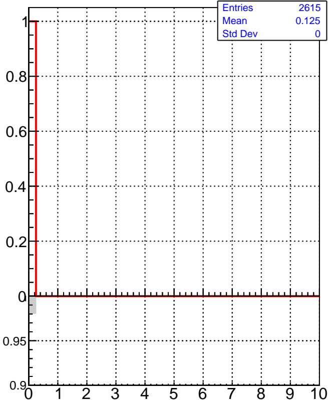
dE/dx estimator 2
