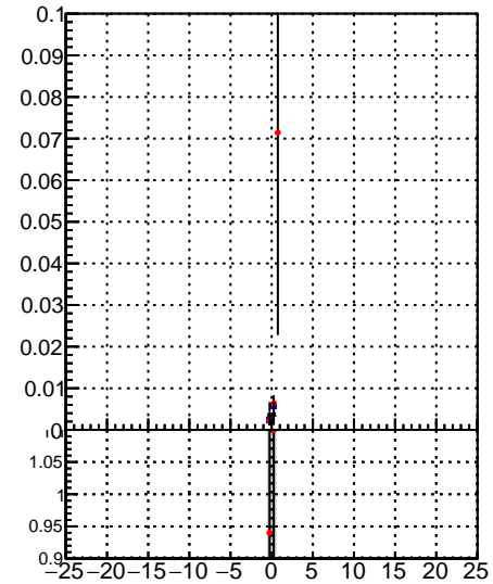
Fake rate vs d trackingIters01-03fac7e 00b trackingLST-Iters01-03fac7e
