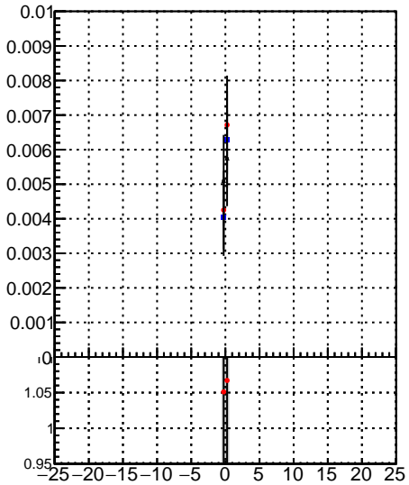
Fake rate vs d trackingLST-Iters01-03fac7e 00b trackingLST-Iters01-03fac7e
