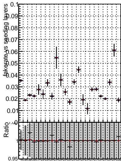
Fake rate vs. ■ DQM ttbarPU mkFit 5iter ● DQM ttbarPU mkFit 5iter updatedPR111 update × DQM ttbarPU mkFit 5iter updatedPR111 update fixPropagation
