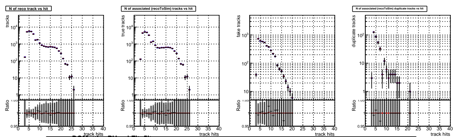
N of reco track vs hit 5 layer 25 layer 50 layer 75 layer 100 layer
