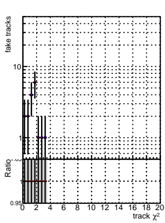
N of reco track vs. DGM ttbarPU mkFit Siter updatedPR111_update fixPropagation DGM ttbarPU mkFit Siter updatedPR111_update DGM ttbarPU mkFit Siter updatedPR111_update
