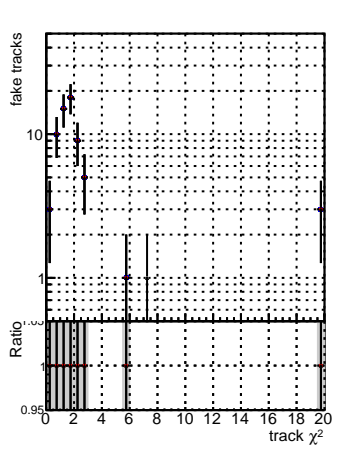
N of reco track vs. \chi^2 BGM ttbar PU mkFit Siter updatedPR11 update fixPropagation
