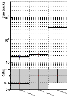
N of reco track vs. DGM ttbarPU mkFit Siter updatedPR111 update fixPropagation DGM ttbarPU mkFit Siter updatedPR111 update
