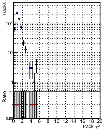
N of reco track vs. DGM ttbarPU mkFit Siter updatedPR111 update fixPropagation DGM ttbarPU mkFit Siter updatedPR111 update
