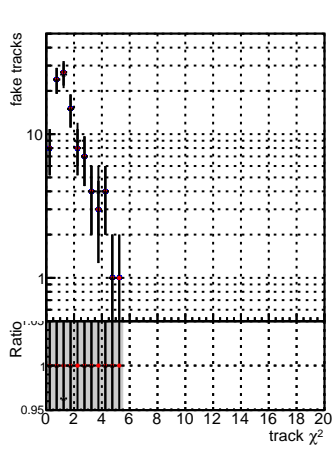
N of reco track vs. DGM tBar PU mkFit Siter updatedPR11 update fixPropagation
