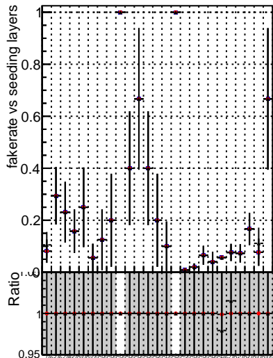
Fake rate vs. — DQM ttbarPU mkFit 5iter — DQM ttbarPU mkFit 5iter updatedPR111 update — DQM ttbarPU mkFit 5iter updatedPR111 update fixPropagation
