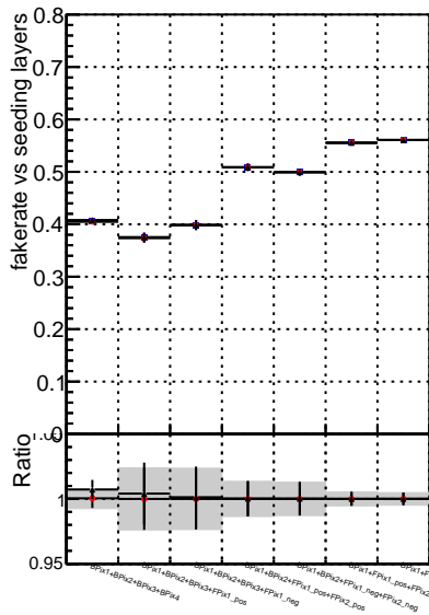
Fake rate vs. — DQM ttbarPU mkFit_5iter — DQM ttbarPU mkFit_5iter updatedPR111_update — DQM ttbarPU mkFit_5iter updatedPR111_update fixPropagation
