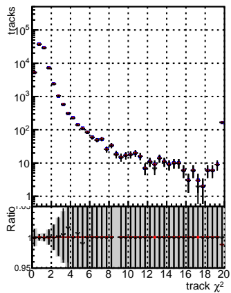
N of reco track vs. —●— BGM ttbarPU mkFit Siter updatedPR111 update fixPropagation —■— BGM ttbarPU mkFit Siter updatedPR111 update fixPropagation —▲— BGM ttbarPU mkFit Siter updatedPR111 update fixPropagation —◆— BGM ttbarPU mkFit Siter updatedPR111 update fixPropagation
