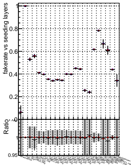
Fake rate vs. ■ DQM ttbarPU mkFit 5iter updatedPR111 update ■ DQM ttbarPU mkFit 5iter updatedPR111 update ■ DQM ttbarPU mkFit 5iter updatedPR111 update fixPropagation
