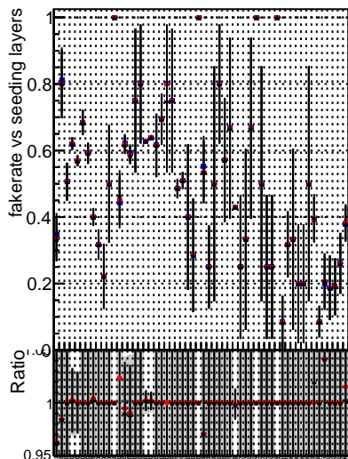
Fake rate vs. — BQM — ttbarPU — mkFit — 5iter — iter updated — PR111 update — update — fixPropagation
