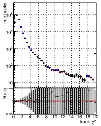
N of reco track vs. \chi^2 for BGM ttbar PU mkFit Siter updatedPR111 update fixPropagation
