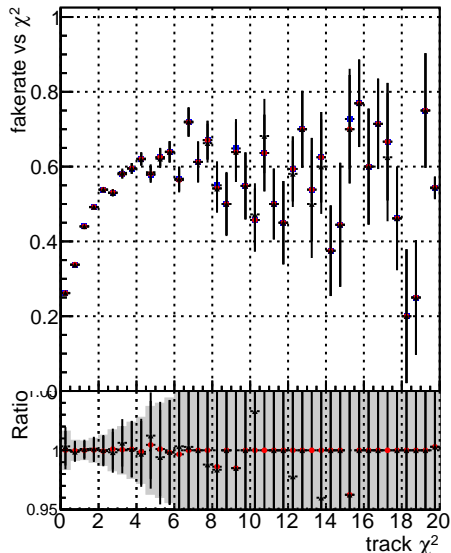
Fake rate vs. — BQM ttbarPU mkFit_5iter — BQM ttbarPU mkFit_5iter updated — BQM ttbarPU mkFit_5iter updated PR111 — BQM ttbarPU mkFit_5iter updated fixPropagation
