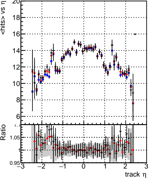
mean hits <math>\langle \text{hits} \rangle \text{ vs } \eta</math>
