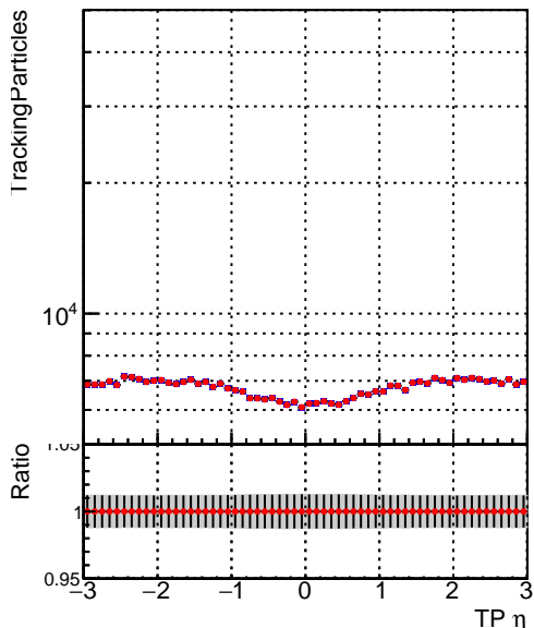
—■ SoftQCD_default —● SoftQCD_ckfPixelLessStep
