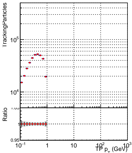
—■ SoftQCD_default —● SoftQCD_ckfPixelLessStep
