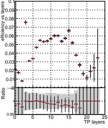
SoftQCD_default SoftQCD_ckfPixelLessStep
