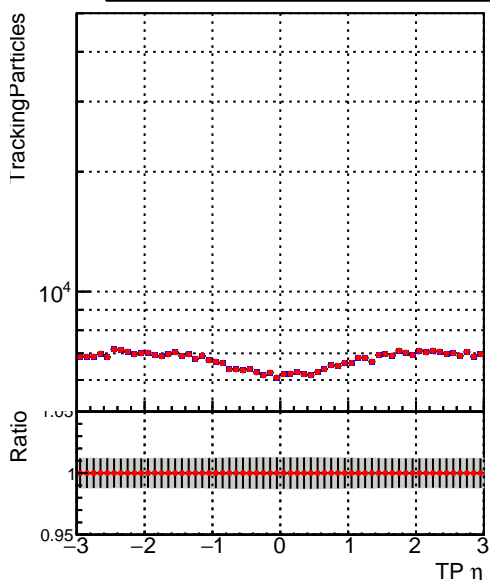
■ SoftQCD_default ● SoftQCD_ckfPixelLessStep
