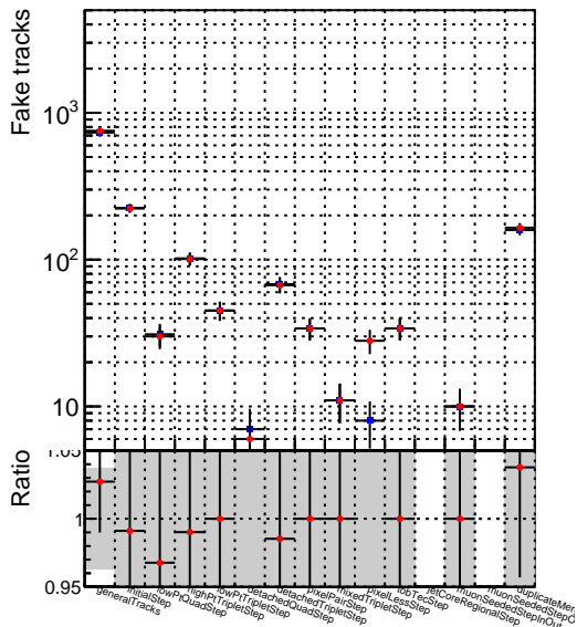
■ SoftQCD_default ● SoftQCD_ckfPixelLessStep
