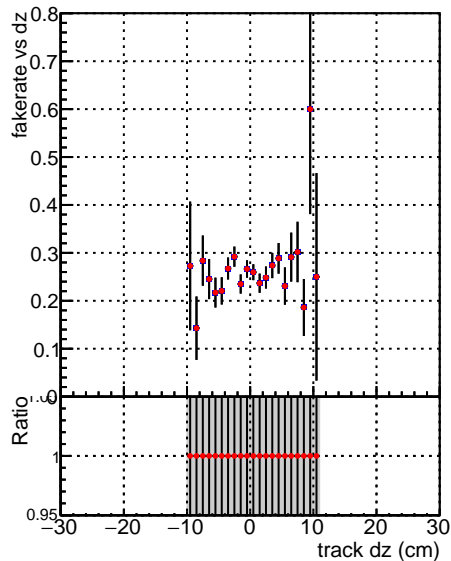
—●— SoftQCDC_default —●— SoftQCDC_ckfPixelLessStep
